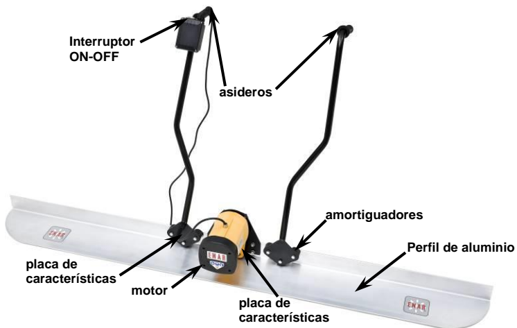
REGLAS VIBRO-EXTENEDORAS CON MOTOR ELÉCTRICO O GASOLINA "QX"
