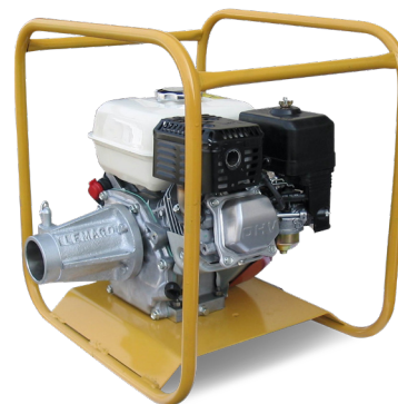
Unidad motriz Gasolina Motor Honda 5,5 HP
